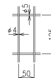
メッシュ寸法図 S=1/5
